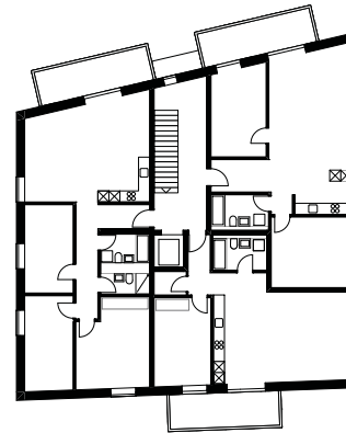
1. Obergeschoss
